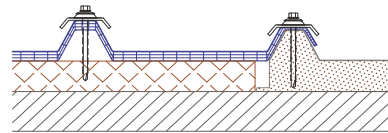
Imbinare laterala cu panou sandwich
